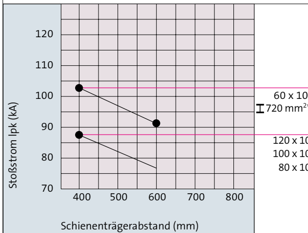
Schienträger Nr. 01 230 185Power
