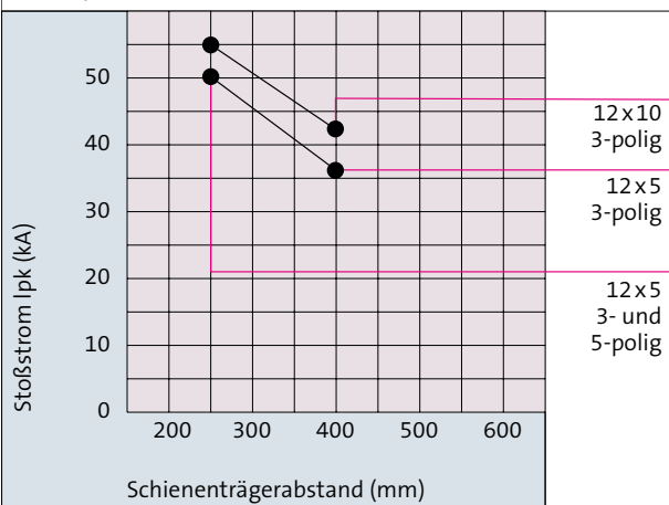
Schienträger Nr. 01 272 30Compact
