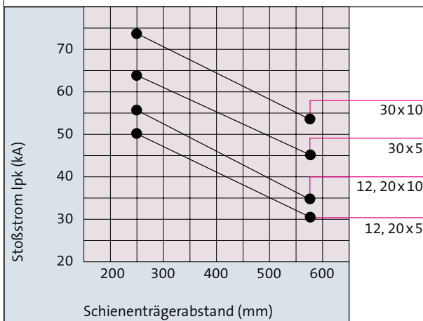
Schienträger Nr. 01 495/01 500/01 315/01 316 60Classic
