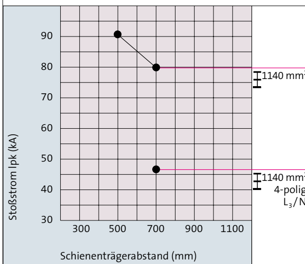
Schienträger Nr. 01 232/01 132 60Classic 2500 A
