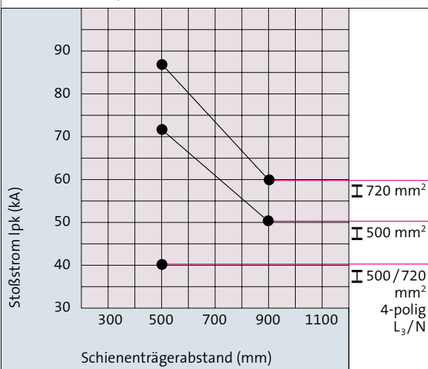
Schienträger Nr. 01 231/01 116, 3- und 4-polig 60Classic 1250 A/1600 A
